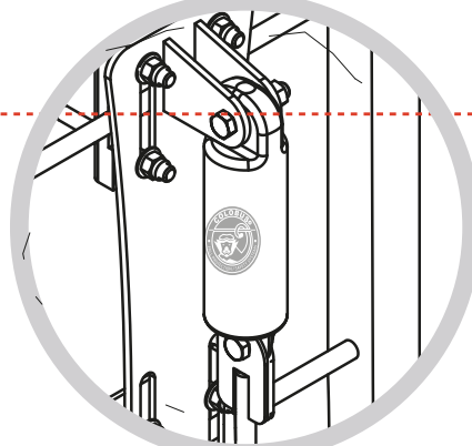
PLACA ACERO INOXIDABLE SISTEMA LÍNEA DE VIDA
